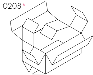
Faltkarton mit integriertem Gefache
