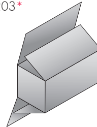
Faltkarton Boden- und Deckelklappen voll überlappend
