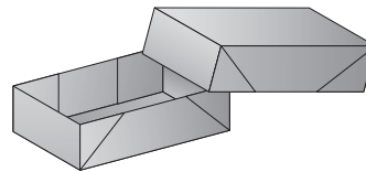
Aufrichtekarton 4 Punkt geklebt, 2-teilig, Boden und Deckel
