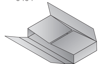
Kreuzverpackung Innenklappen zusammenstoßend 1-teilig oder 2-teilig
